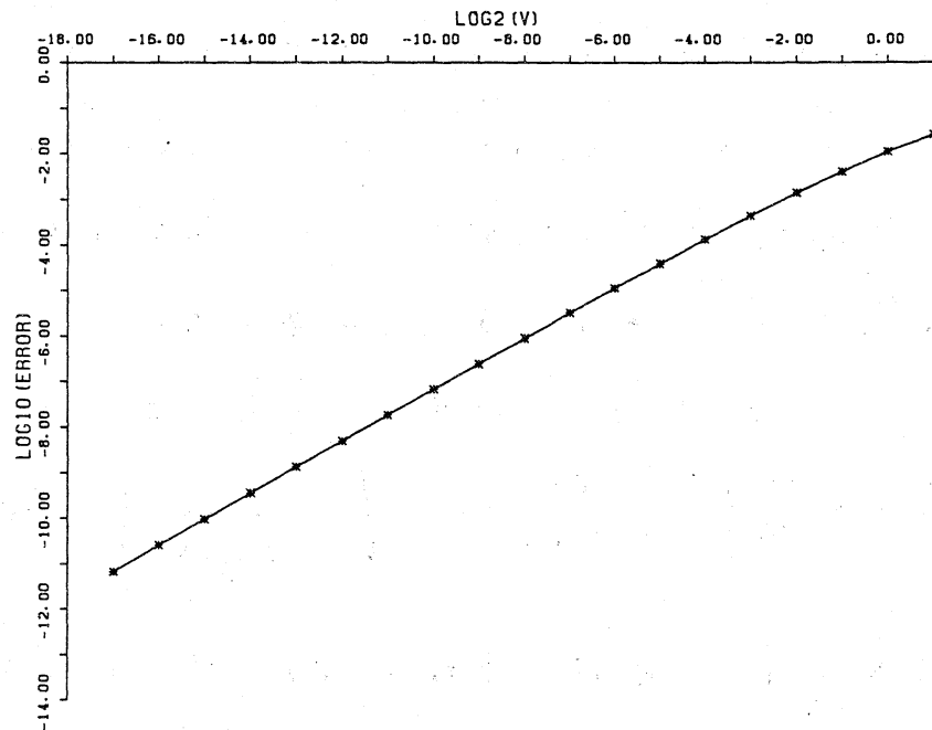
図 1 g_4(v/\sqrt{3}) の誤差
