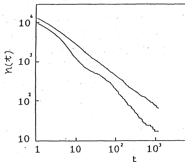
図 1. 1次元 L L V系におけるダイナミックス ( M=40,000 )。初期条件として上の曲線は (n_1 : n_2 : n_3) が (1 : 1 : 1) のときであり、下の曲線は (7 : 2 : 1) のときである。
