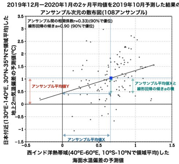
図 4: 2019 年 12 月から 2020 年 1 月の 2 ヶ月平均を対象として、2019 年 10 月初旬から予測を開始した 108 のアンサンブル予測シミュレーションの結果を使ったアンサンブル次元の散布図。縦軸は日本付近(130°E-140°E, 30°N-35°N で領域平均)の地上 2m 気温偏差の予測値で、横軸は、西インド洋熱帯域(40°E-60°E, 10°S-10°N で領域平均)の海面水温の予測値。黒い点が 108 アンサンブルメンバーそれぞれの値で、青い四角がアンサンブル平均値を示す。黒線は線形回帰直線。相関係数は 0.33 で 90%の信頼区間で統計的に有意。回帰直線の傾き a は 0.90 で 90%の信頼区間で統計的に有意。
