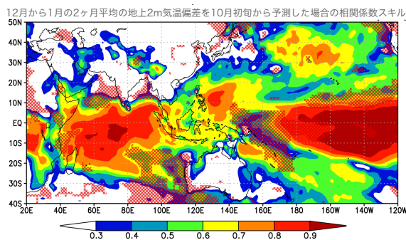
図 1: 12 月から 1 月の 2 ヶ月平均の地上 2m 気温偏差を 10 月初旬から予測した場合の相関係数スキル。1 に近いほど予測スキルが高い。SINTEX-F2 季節予測システム(Doi et al. 2019)による 1983-2015 年の過去再予測実験の結果で、108 アンサンブルメンバーの平均値と NCEP/NCAR 再解析データの値から計算した。Persistent 予測の予測スキル(自己ラグ相関係数)より低い値は赤色で網掛けをした。
