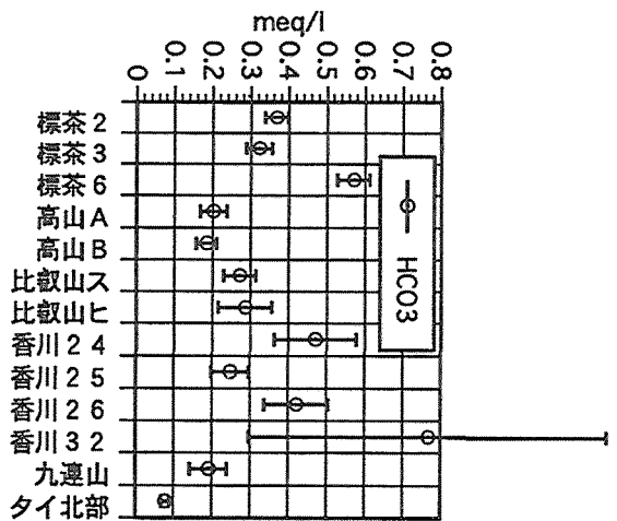
図-3(b) 森林流出水の各イオンの平均濃度と標準偏差
