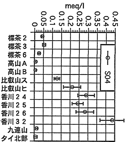
図-3(b) 森林流出水の各イオンの平均濃度と標準偏差
