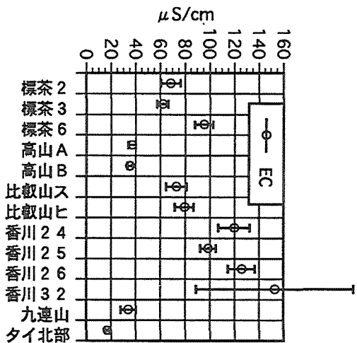
図-3(a) 森林流出水の各イオンの平均濃度と標準偏差
