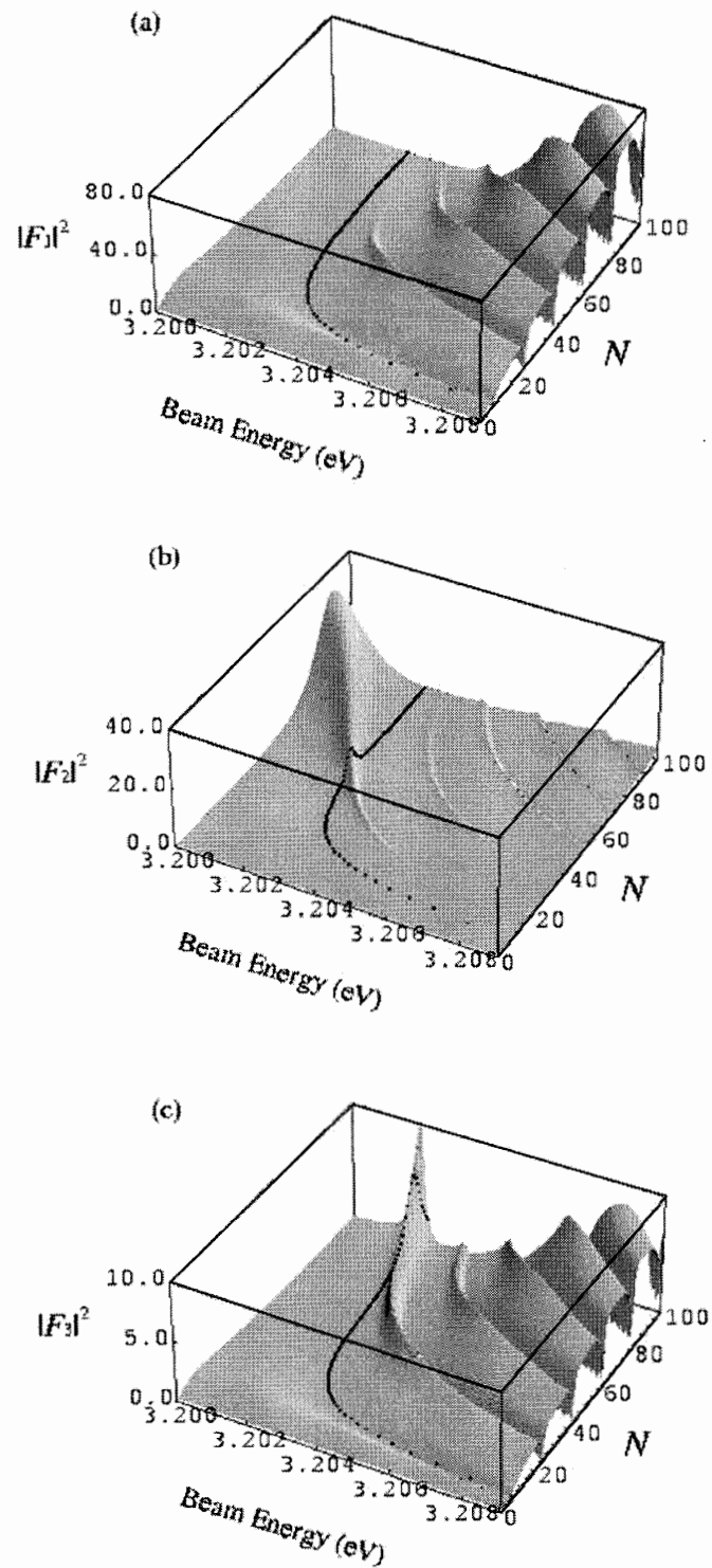
図2 系のサイズ N と入射光エネルギーの関数として表示した内部電場強度. サイズ量子化準位 n = 1, 2, 3 に対応する空間構成成分を別々に表示. 点線はサイズ N とともに変化する n = 1 励起子エネルギーに沿ったこの曲面の切り口. \gamma = 0.06 meV [13]
