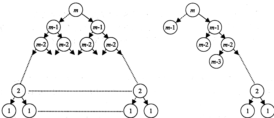
図 4: 2つの方法が構築するネットワークの様子
