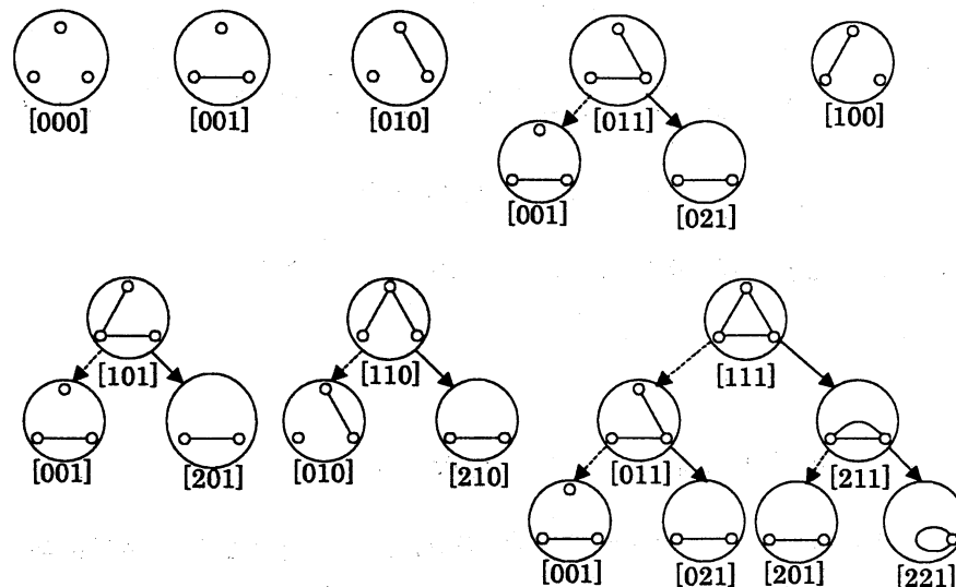
図3: 図1で示したネットワークの全部分ネットワークに対する factoring 法の適用
