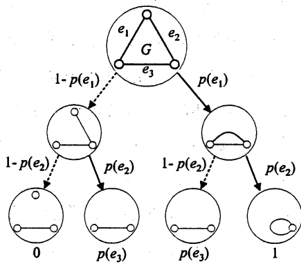
図 1: factoring 法による総合信頼度計算の例
