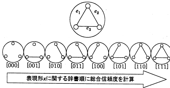
図 2: 図 1 で扱ったネットワークの全部分ネットワークとそれらの表現形
