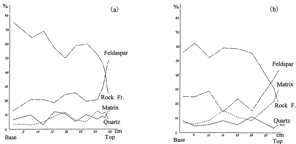
第2図 舞鶴層群タービダイト級化層の砂岩鉱物組成 (a, b 二つの試料の例)。
