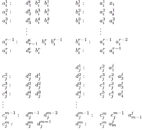
図 1 \mathcal{C}(X, r) の希望リスト
