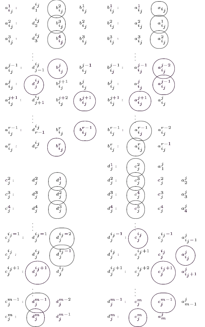
図 2 補題 2.2 の証明で使われるマッチングの一部
