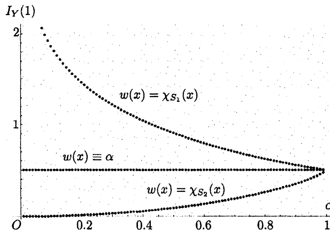
図 6.2 \beta = 0 を満たす荷重関数に対応する I_Y(1) のグラフ
