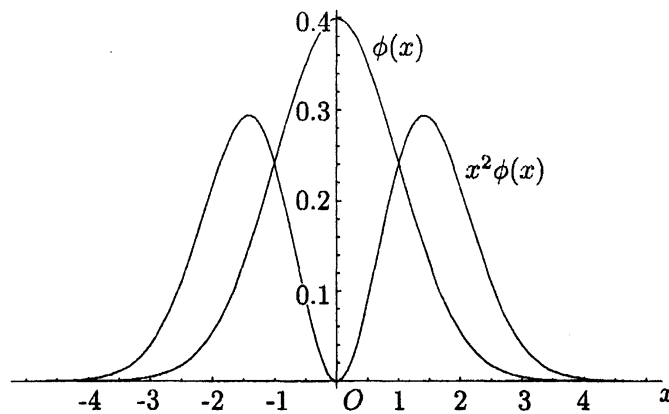
図 6.1 \phi(x) , x^2\phi(x) のグラフ
