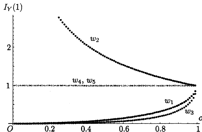
図 6.6 荷重関数の取り方と I_Y(1) のグラフ
