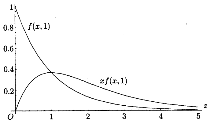
図 6.4 f(x, 1) , xf(x, 1) のグラフ
