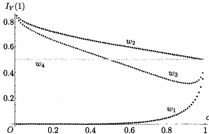
図 6.3 荷重関数の取り方と I_Y(1) のグラフ
