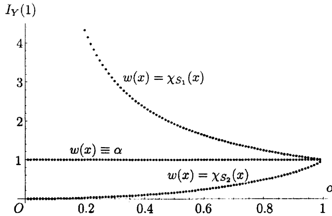
図 6.5 \beta = 0 を満たす荷重関数に対応する I_Y(1) のグラフ
