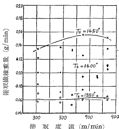
第5圖 T_N=1040^\circ の場合
