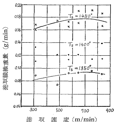
第4圖 T_N=1020^\circ の場合
