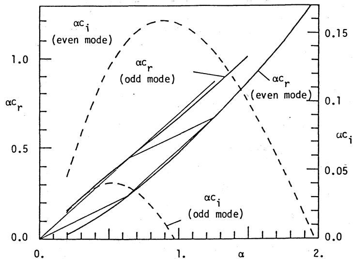
図1. 二次元ジェットの線形固有値. R=1000 . 実線は \alpha c_r 、破線は \alpha c_i を表す.
