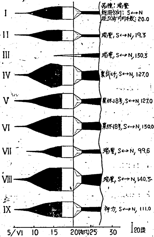
第2図 昆虫総量の消長(本図にはデラ颱風の影響が出ています) 径30cm 捕虫網による10回宛の定量的調査, 各区共中央附近の2~5 短冊使用 (1949)。
