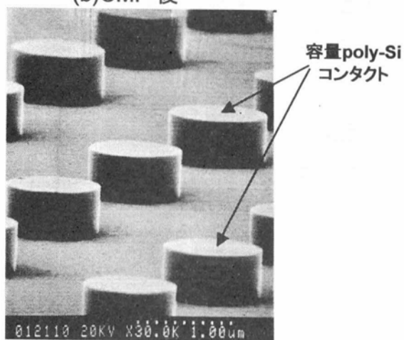
(c) (b)から試験的に SiO 2 を除去した後
