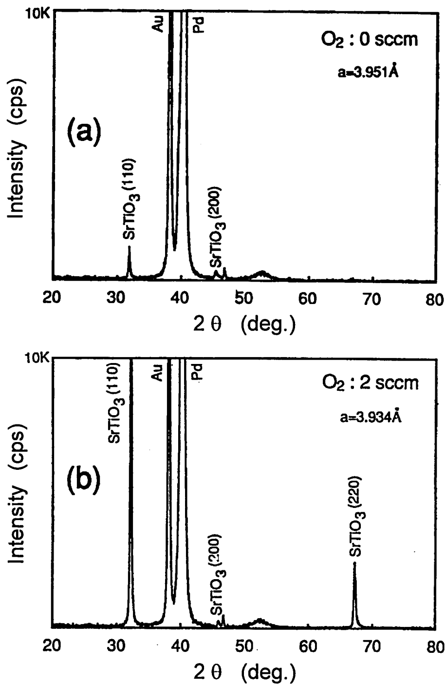
図 2.3 成膜中に \text{O}_2 ガスを流した場合と流さなかった場合の \text{SrTiO}_3 薄膜の XRD パターン
