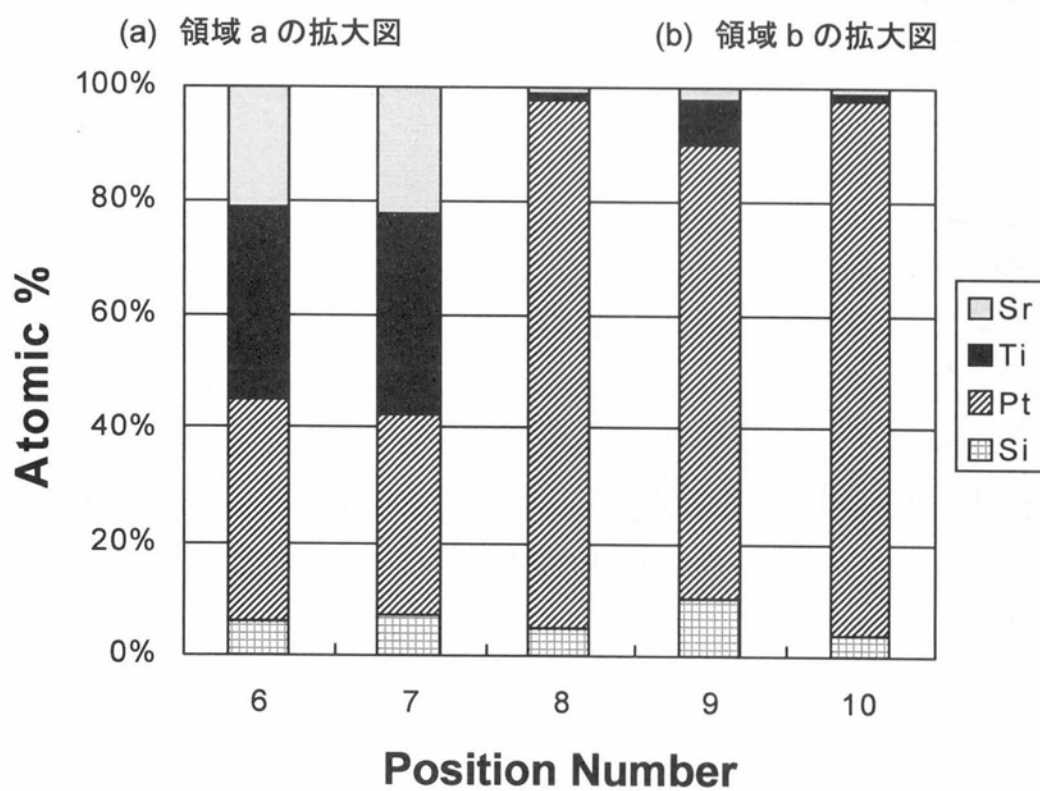
(c) 分析結果
