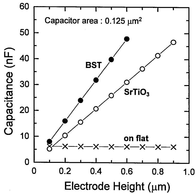
図 4.31 1GbDRAM に必要な単純スタック型電極の高さ
