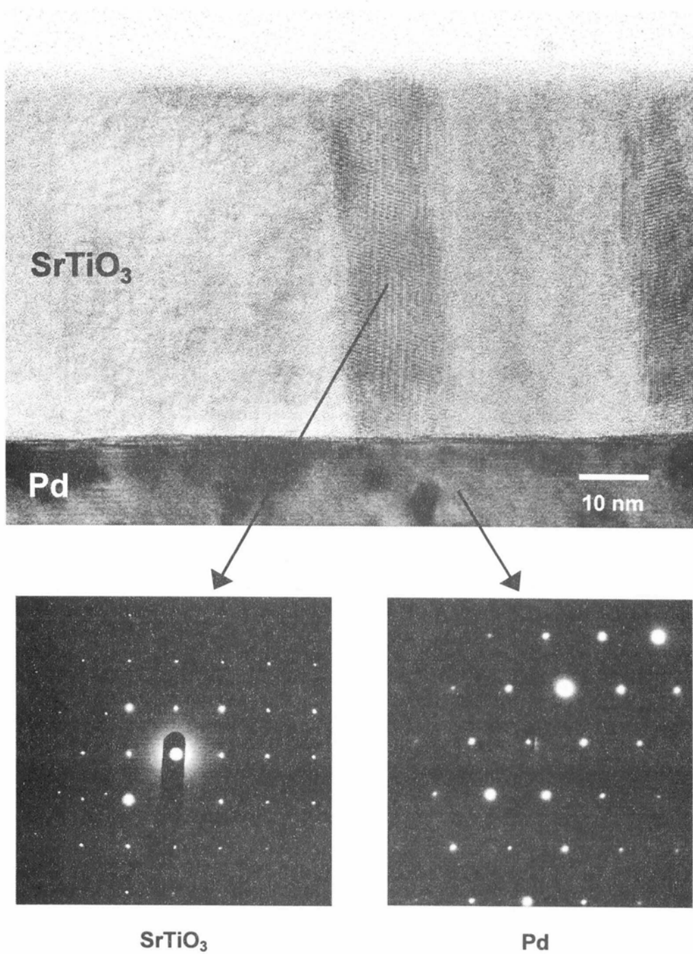
図 2. 15 基板温度 540 °C で作製した \text{SrTiO}_3 薄膜の 断面 TEM 写真と電子線回折パターン
