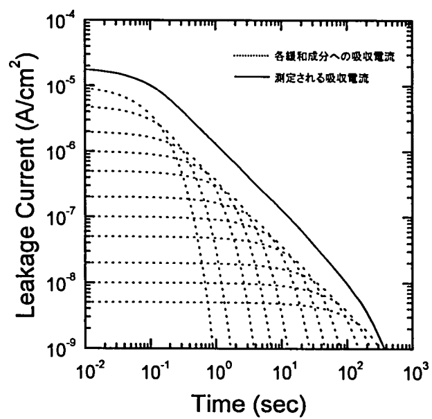
図 2.48 Curie - von Schweidler 則による吸収電流
