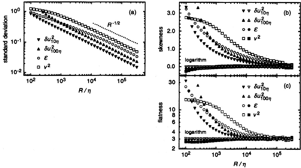
図 2: \delta u^2_{10\eta R, R}/u^2_{K, R} , \delta u^2_{100\eta R, R}/u^2_{K, R} , \epsilon_R , v_R^2 の統計. (a) 平均値で規格化した標準偏差. (b) Flatness. (c) Skewness. 横軸は R/\eta .
