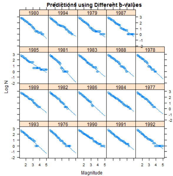
Fig. 5. Linear fit using different parameter values.
