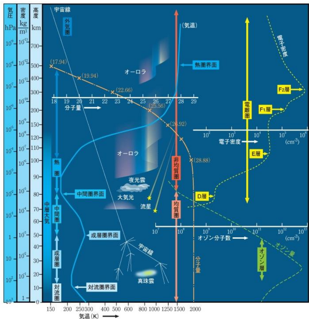
図 1：高度 700km 以下における大気の流れ・密度・温度・大気の大平均分子重量の变化。右側にはオゾンの高度分布と電離圏の電子密度も示している。 1)
