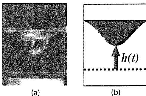
図 2: 実験例: (a) は実験例の写真であり、(b) は (a) の模式図である。(b) における黒色部分は渦を表している。また (b) における点線を底とし、矢印のように h(t) を定める。
