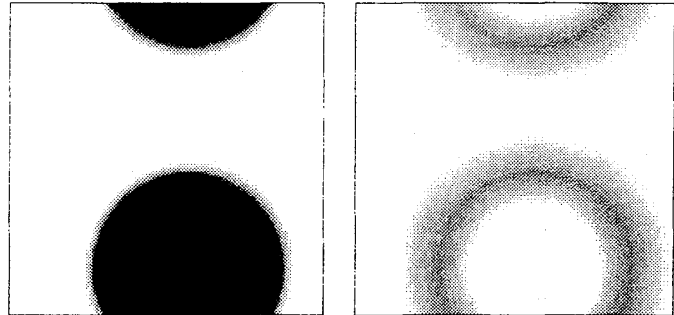
(a) A セグメント濃度 \phi_{AB,A}(\mathbf{r}) + \phi_A(\mathbf{r}) (b) AB ジブロックコポリマー濃度 \phi_{AB,A}(\mathbf{r}) + \phi_{AB,B}(\mathbf{r})
