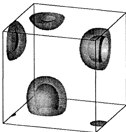
図 32: AB ジブロックコポリマー / A ホモポリマーブレンドのシミュレーション結果。灰色の面は \chi_{AB,B}(\mathbf{r}) = 0.5 の等値面を表す。
