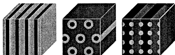
図 3: トリブロックリニアコポリマーの形成するマイクロ相分離構造の一例。黒、薄い灰色、灰色の部分はそれぞれ異なるブロックを表す。
