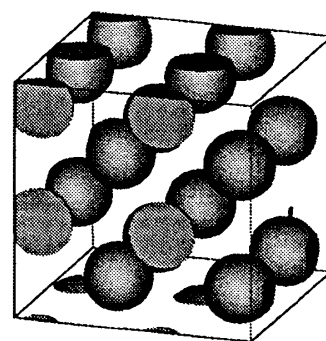
図 21: AB ジブロックコポリマーメルトのシミュレーション結果。灰色の面は \phi_A(\mathbf{r}) = 0.5 の等値面を表わす。
