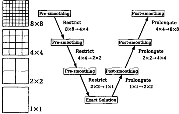
図 37: V サイクルの概念図。最も細かい格子が 8 \times 8 の 2 次元系の場合。この場合、 8 \times 8, 4 \times 4, 2 \times 2, 1 \times 1 の 4 種類の格子を用いる。最も粗い格子上では厳密解が得られる。
