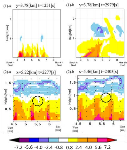
Fig. 10 Buoyancy
