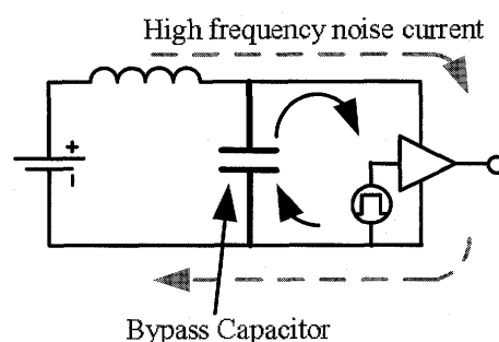
第2図 バイパスコンデンサの役割
