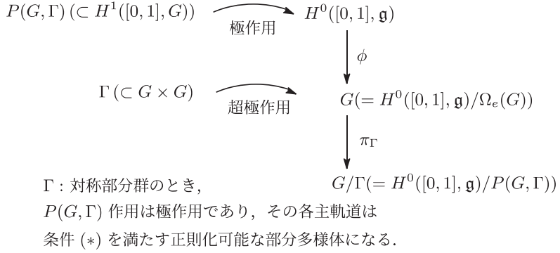
図 6.1 : ヒルベルト空間上の極作用の例
