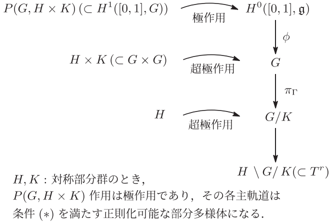
図 6.2 : ヒルベルト空間上の極作用の例 (続)
