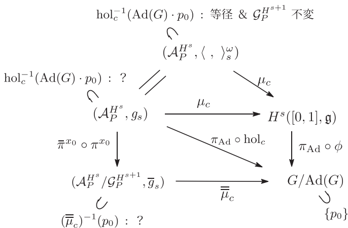
図式 9.2 : G 内の随伴軌道からえられる \mathcal{G}_P^{H^{s+1}} 不変な等径部分多様体
