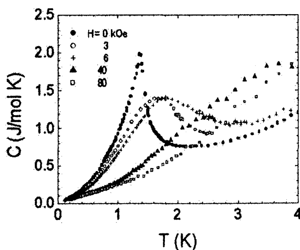
図 2 比熱の温度依存性の磁場変化
