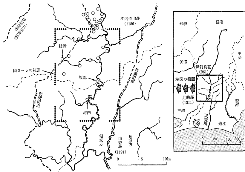
図1 対象山域と周辺の諸領域
