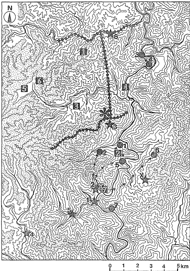
図5 坂部のステージ (1428頃～1495)
