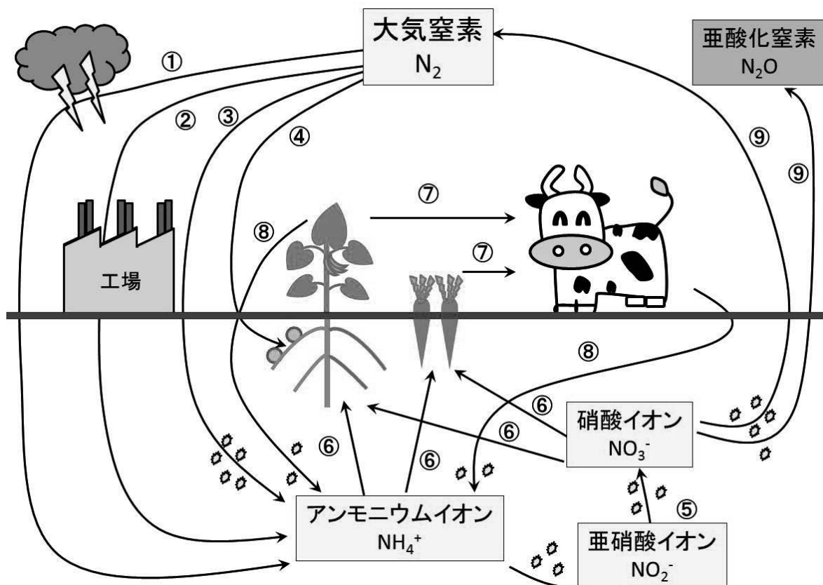
図1 生存圏における窒素循環
