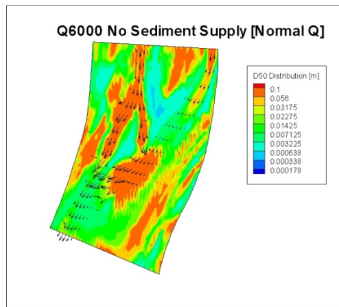
Fig. 16 D50 [m] (Case No.1)
