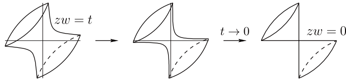
図 2: 複素双曲線 zw = t の族 ( t \in \mathbb{C} はパラメータ). この図の“実断面”が図 1。
