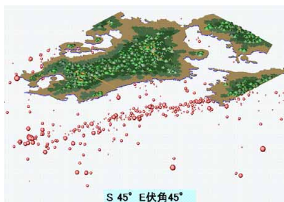
図2 3D日向灘地震震源分布図
