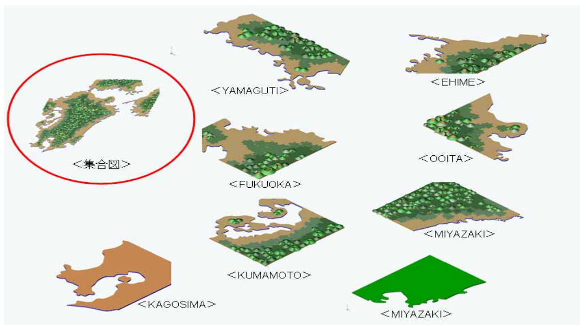
図3 九州全域の8区域分解図
