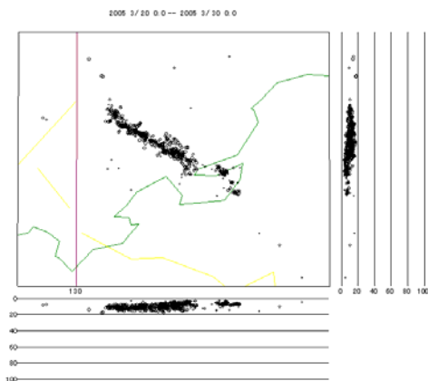
図 5 2 次元震源分布図
