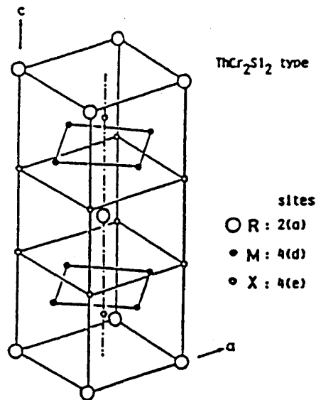
Fig.1 \text{DyRu}_2\text{Si}_2 の結晶構造
