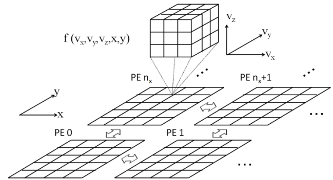
図 1 5 次元 Vlasov コードにおける空間領域分割[8].
