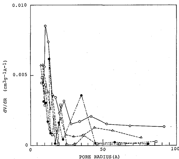
Fig. 3. Pore size distribution curves of the gels aged for 30 days at 40°C. [\text{HCl}]/[\text{TMOS}] = 0.10 (—○—), 0.15 (---△---), 0.20 (---□---) and 0.25 (---●---).
