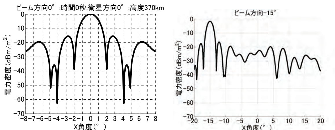
図 10.2.2.3 ビームパターンの理論値
