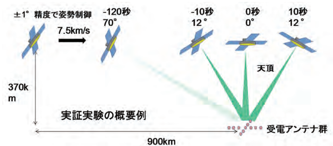
図 10.2.2.1 SPS のための小型電力試験衛星実験シーケンスの例
