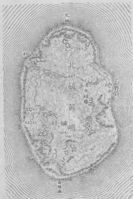
(一ノ分万五) 島 黄 硫 北
