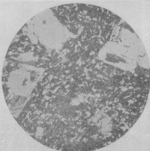
北硫黄島の輝石
