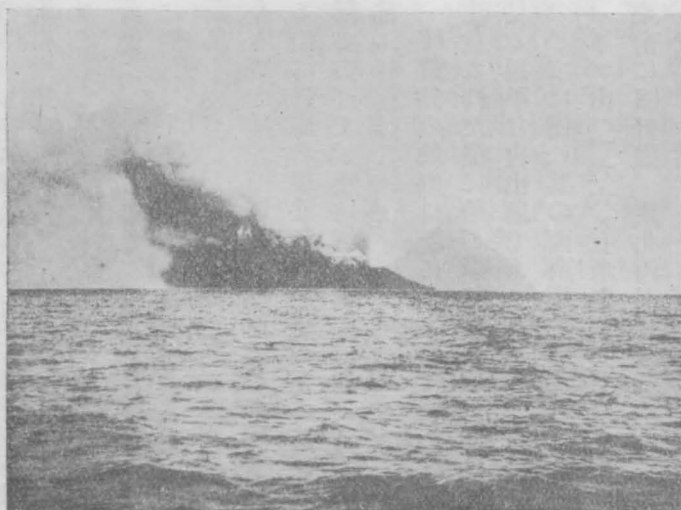
新硫黄の噴煙
