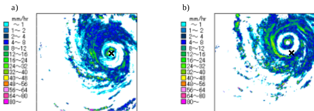
第3図 台風0314号のレーダーエコー。xは宮古島の位置を示す。
