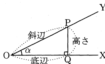
図4. 三角比の定義 (修正版)
