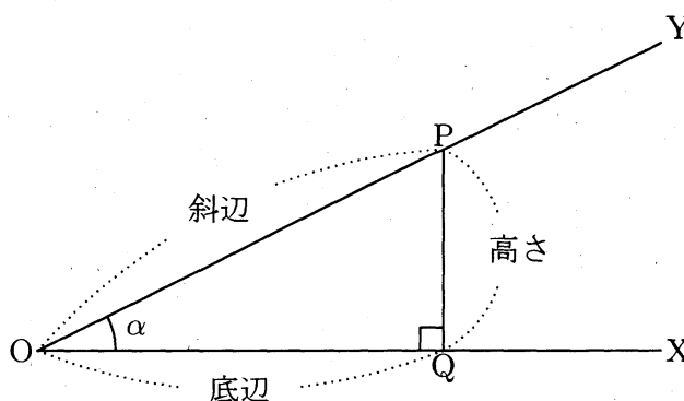
図5. 三角比の定義 (修正版) の拡大図
