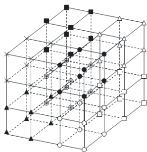
図 4 ブロックマルチカラーオーダリングの例 ( l_x = l_y = l_z = m_x = m_y = m_z = 2 )
