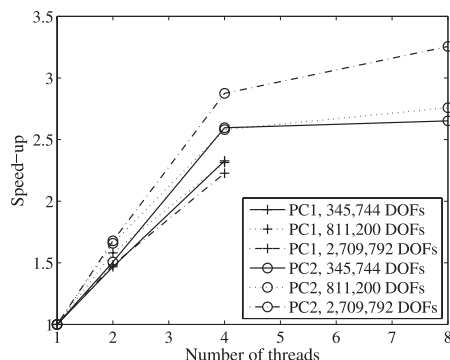
図 8 速度向上率 (テストモデル 1)
