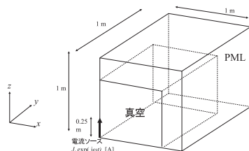
図 5 テストモデル 1 Fig. 5 Test model 1.
