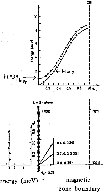
図 19. \text{CsNiF}_3
