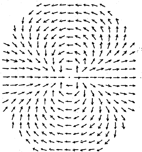
q=2 の渦
