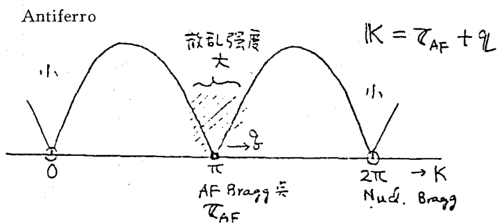
図 6. TMMCのスピンドYNAMICKS
