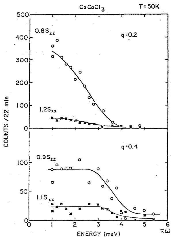
図 48-2 実測された profile. 図 48-7 の右半分 \hbar\omega > 0 に対応する。
