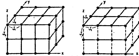
(c) 1次元磁性体 ( J_1 \gg J_2, J_3 ) (d) 分子型磁性体 ( J_1 \gg J'_1, J_2, J_3 )
