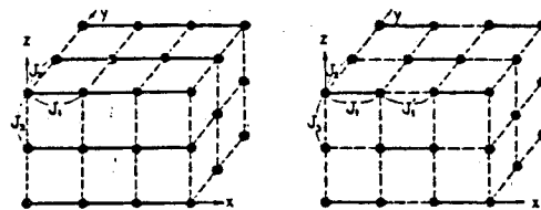
図1. 3次元から低次元へ, 黒丸はスピン格子点を示し, 実線は強い相互作用, 点線は弱い相互作用を示す。
