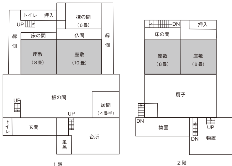
図3 家屋構造
