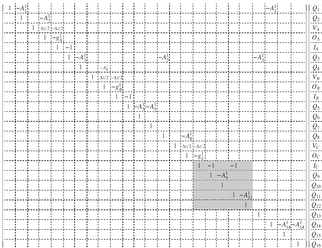
図-4 複数ダムが存在する場合の状態方程式の係数行列 X_i と状態ベクトル Q_i ：灰色部分はダム C に関連する部分係数行列 X_C 値が何も入ってない成分は 0 である。
