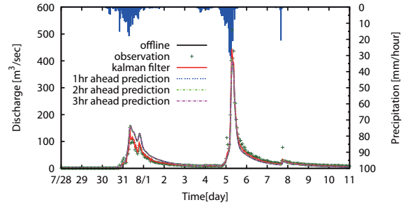
(a) 流入量（点線は洪水調節開始流量）
