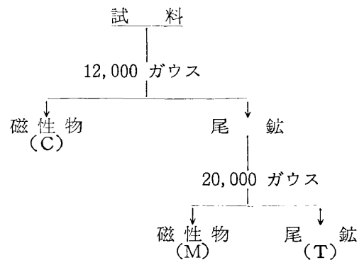
図 3 磁選の方式
