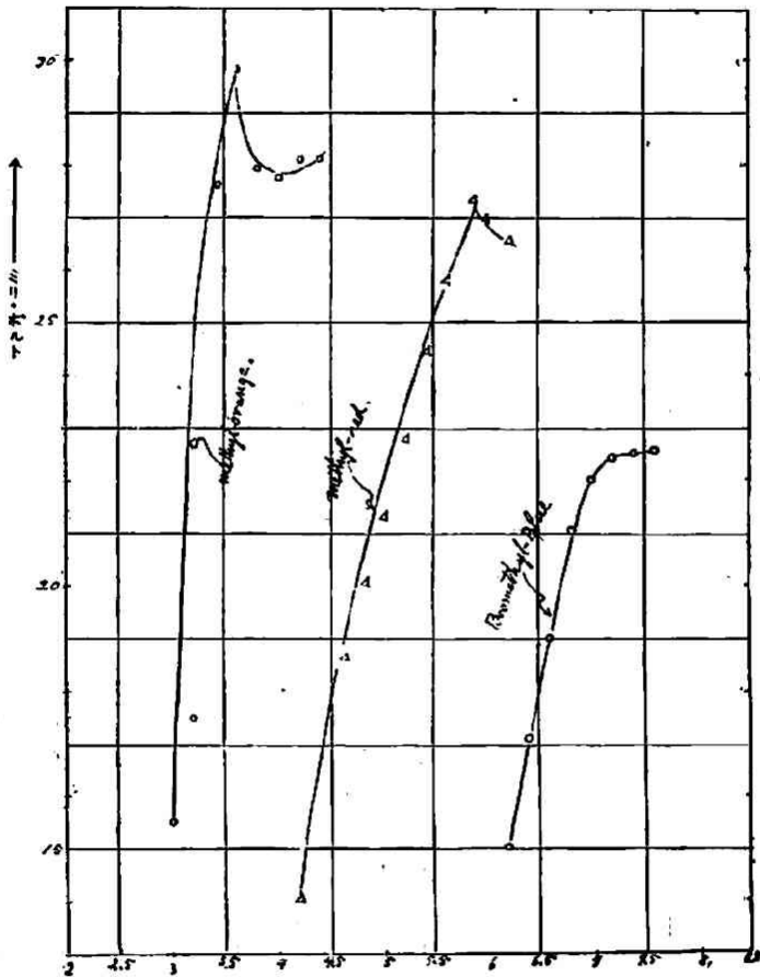
第十二図 指ひ薬と酸化銅電極の Becquerel 効果との関係
