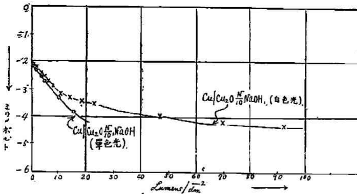
第八圖 光の強さと \text{Cu/Cu}_2\text{O} \frac{N}{10} \text{NaOH} 電極との関係
