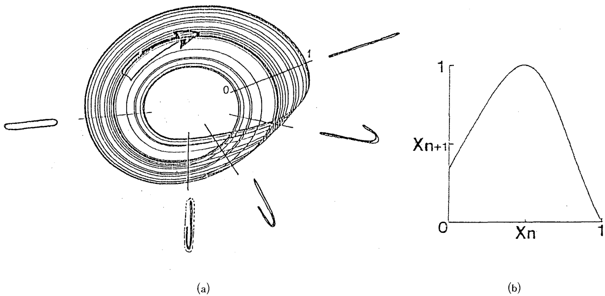
第7図 (a) Rösslerアトラクタ及び各Poincaré断面で見たアトラクタの切り口。 (b) 対応する近似的一次元写像。
