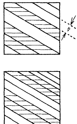
第15図 Hénonアトラクタを粗さ \eta の格子を通して見れば3本の線に見えたり(上図), より小さな \eta をとれば(下図)4本に見える。
