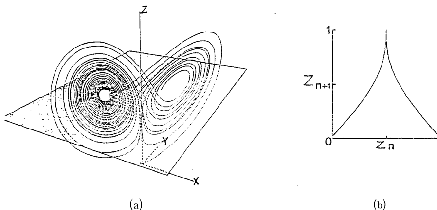
第6図 (a) Lorenzアトラクタ(D. Ruelle, La Recherche 11 (1980)132による)。 (b) 対応する近似的一次元写像。
