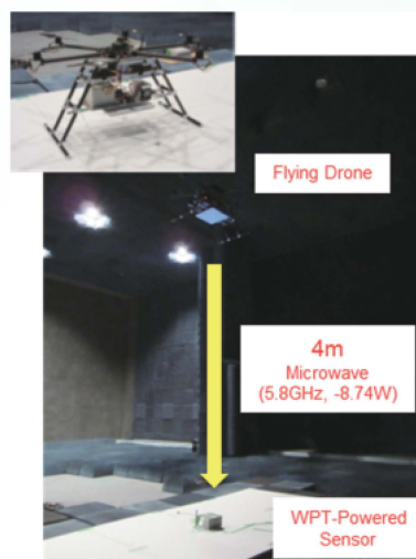
(写真2) 2015年に生存圏研究所で行ったドローンからのマイクロ波ワイヤレス給電センサーの実験
