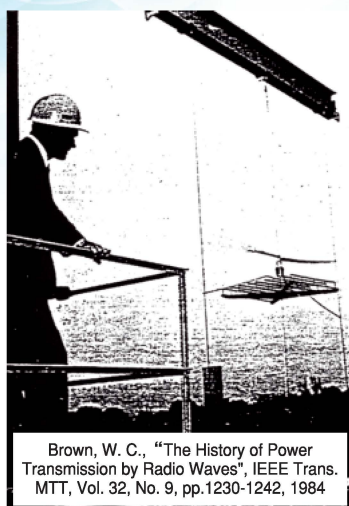
(写真1) 1964年にアメリカで行われたドローンへのマイクロ波ワイヤレス給電実験
