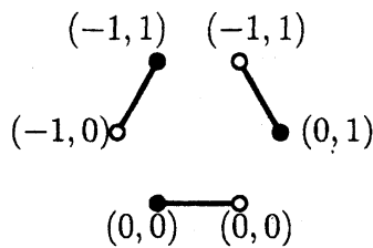
図 3: 正六角形
