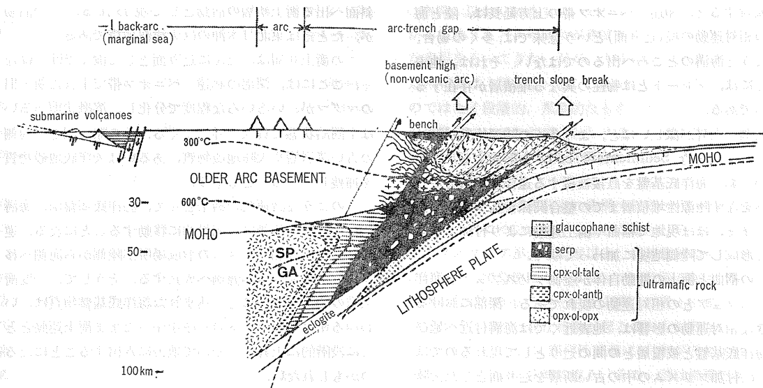
第17図 二畳～三畳紀における黒瀬川構造帯. 丸山 (1978)
