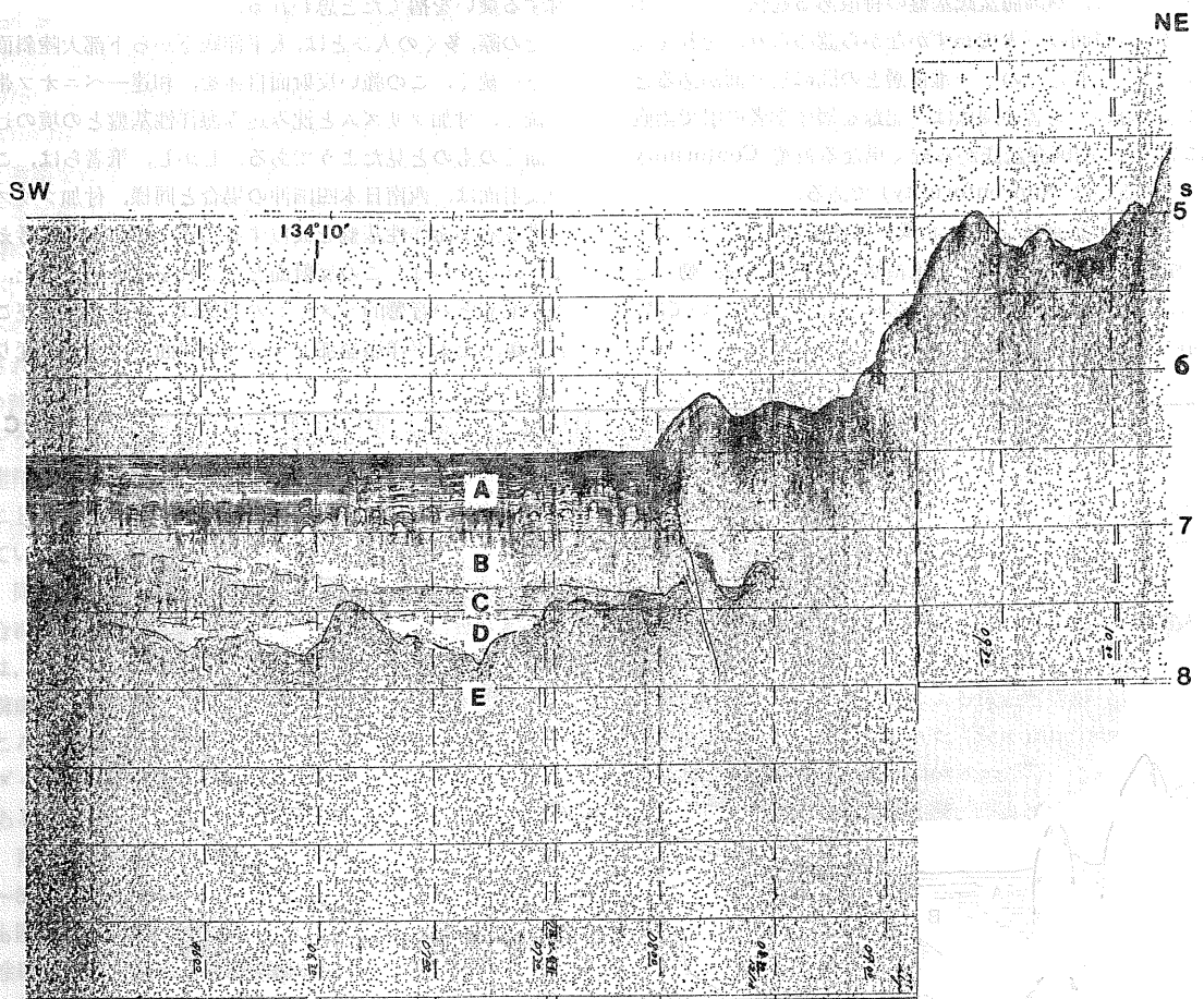
第10図 四国南方の反射法音波探査断面
