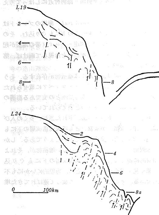
第3図 三陸沖の反射法音波探査断面解釈図。 HONZA (1977) に一部加筆
