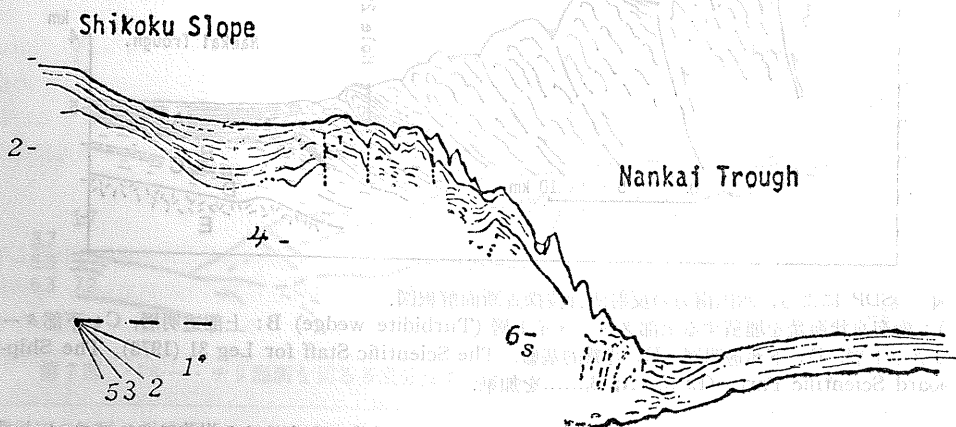
第2図 四国南方の反射法音波探査断面解釈図。井上ほか (1977)、奥田ほか (1974) より
