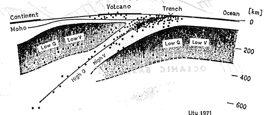
第14図 日本付近における上部マントルの構造と深発地震面模式図。UTSU (1971)
