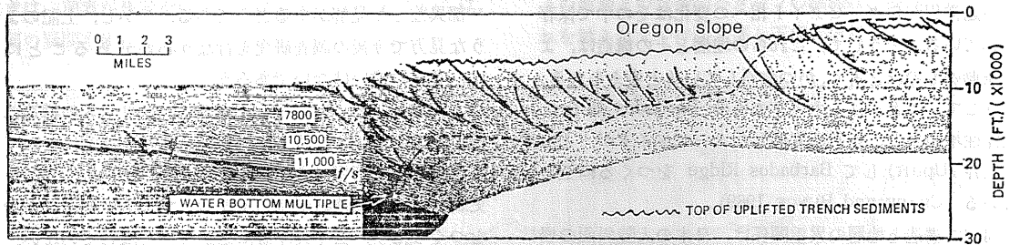
第6図 オレゴン沖の大陸斜面を切る多成分反射法音波探査断面. KULM and FOWDER (1975) より
