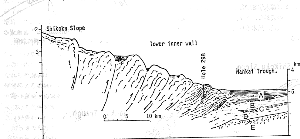
第4図 DSDP による、四国南方の反射法音波探査断面解釈図。
