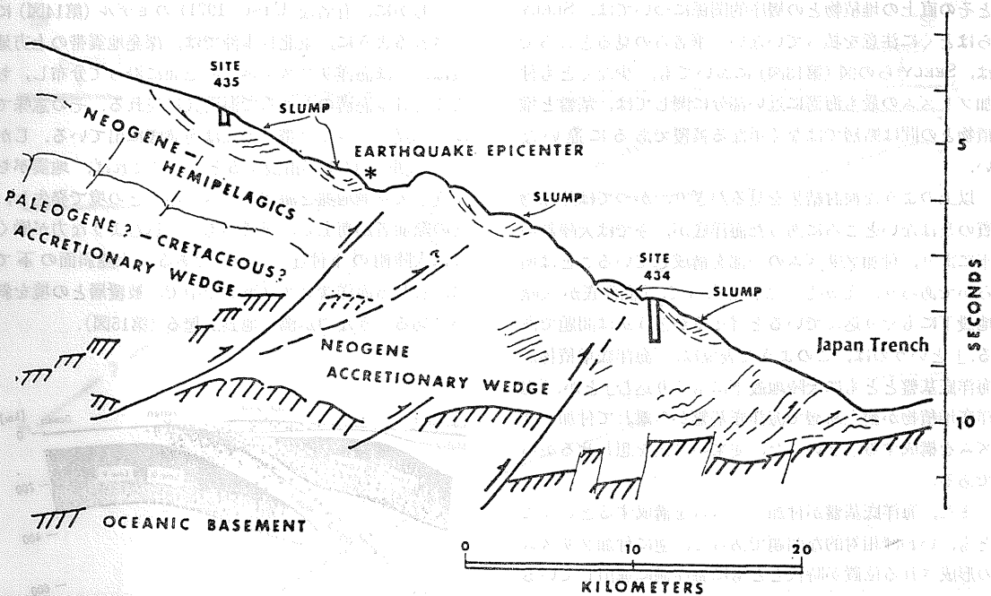
第12図 IPOD 事前調査, 三陸沖多成分反射法音波探査断面解釈図 Scientists aboard Glomer Challenger for Leg 56 (1978)
