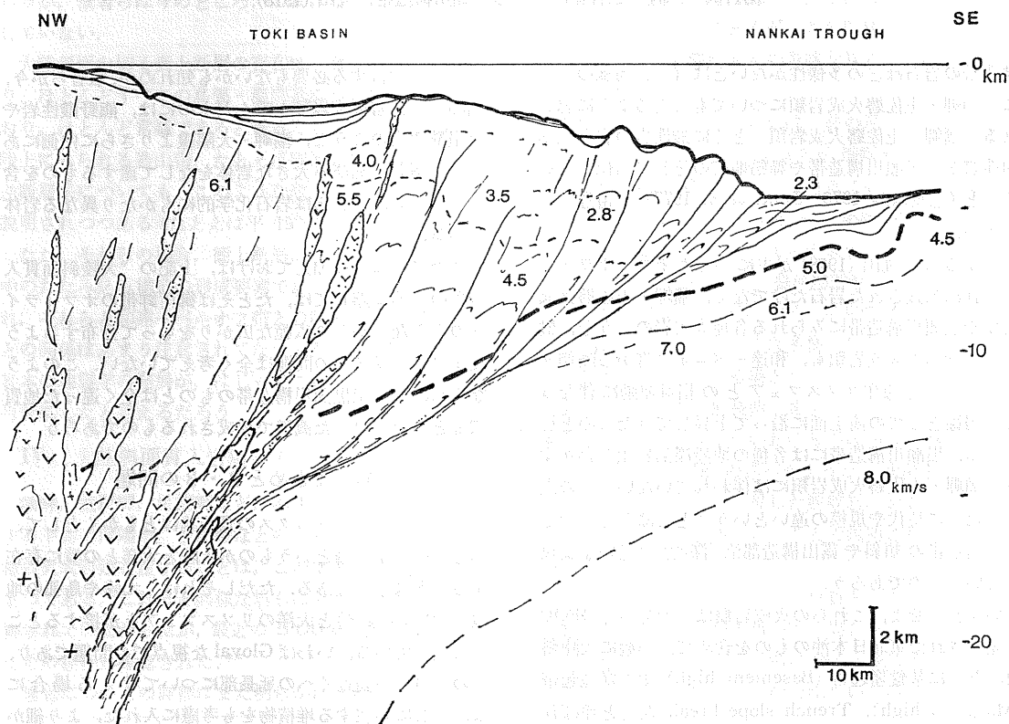
第18図 四国南方の大陸斜面-南海舟状海盆を切る地殻断面模式図。
