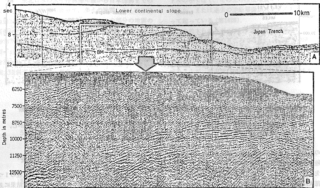
第11図 東北日本三陸沖下部大陸斜面 - 日本海溝を切る多成分反射法音波探査断面, Beck et al. (1975) 太平洋底の基盤の反射が下部大陸斜面 (陸側海溝斜面) の下へ続いている。
