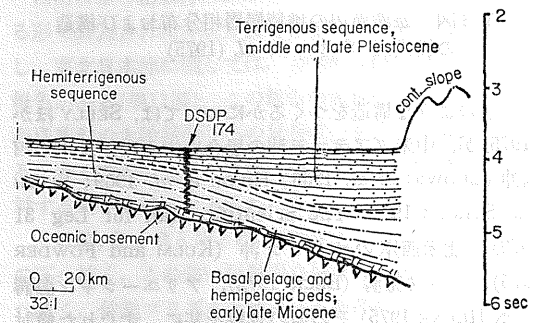
第5図 オレゴン沖 Turbidite wedge の反射法音波探査断面解釈図. VON HUENE and KULM (1973) より, SCHOLL (1975)。
