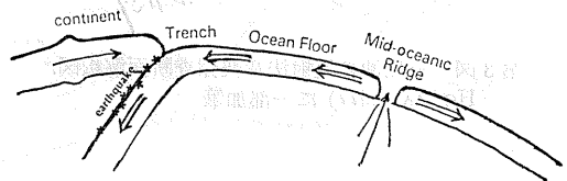
第1図 海洋プレートの“Subduction”と地震の発生、模式図。HOLMES (1978) の図に加筆
