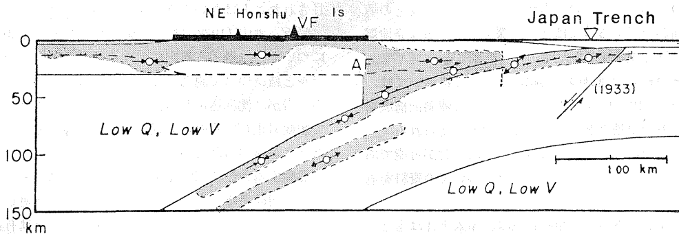
第15図 東北日本の地殻・上部マントル構造の模式図
