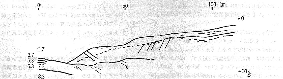
第7図 ペルー・チリ海溝を切る多成分反射法音波探査断面解釈図. HUSSONG et al. (1976)
