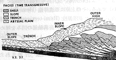
第8図 海溝周辺の堆積層層相分布および構造の模式図. SEELY et al. (1975)
