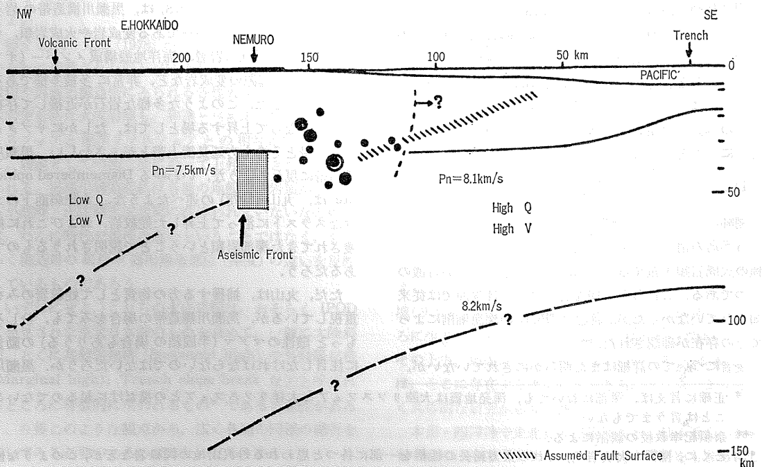
第16図 1973年根室沖地震の震源(丸印)を示す断面図(海溝軸に直角)。鈴木・岡田(1977)。 推定断層面の位置に注意
