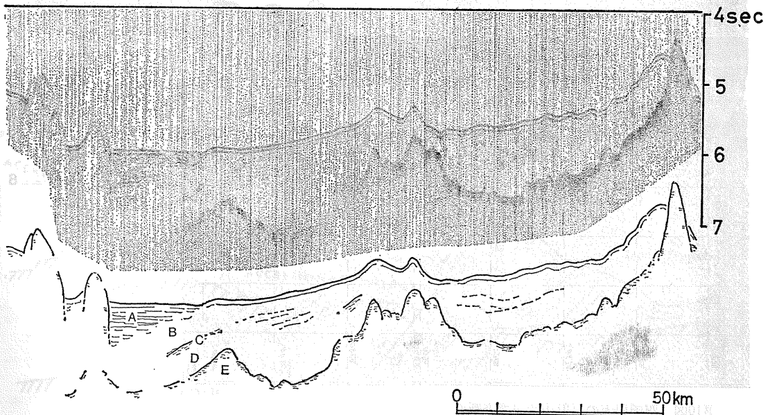
第9図 潮岬南方の反射法音波探査断面と解釈図 四国海盆・南海舟状海盆の音響的基盤の起伏状態が、図の左側で大陸斜面構成物の下へ続く気配が見える。三沢(1967)
