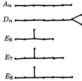
Dynkin Diagram
