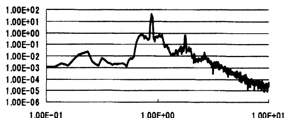
図6：不規則擾乱 (Bredschneider spectrum) と規則波における側帯擾乱の成長；水槽実験
