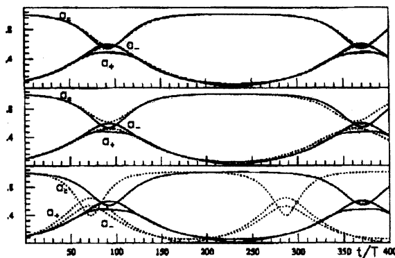
図4： 弱非線形解と完全非線形解との比較。 BF 不安定波列の長期発達
