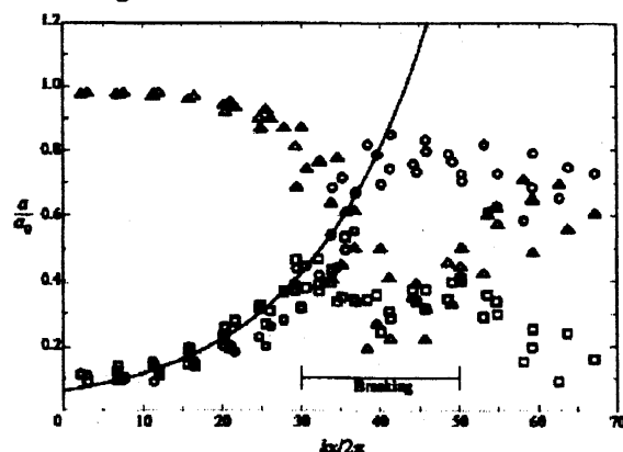
図 3: 中心波 (三角) と側帯波 (丸、四角) の振幅の発達。碎波以降、低周波側の側帯波 (丸) のエネルギーが高い (Tulin & Waseda)
