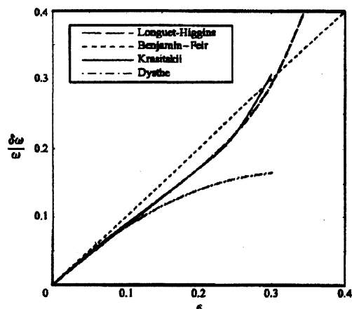
図 2: 各初期相度における最大成長率となる初期相度とバンド幅の組み合わせ。Waseda & Tulin (1999) より抜粋。
