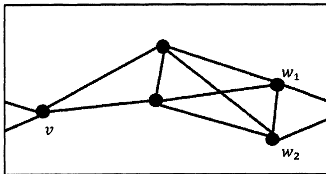
図 7 G と l の交差が複数あり同一のノードとつながっている例
