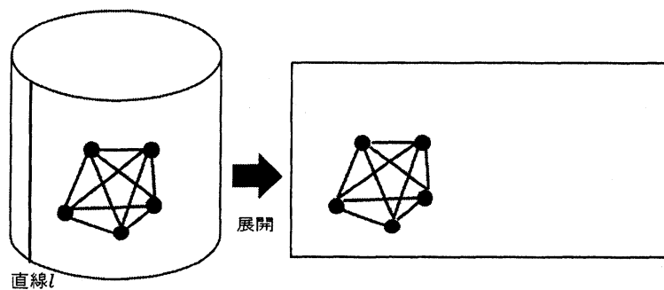
図 5 グラフ G と直線 l の例
