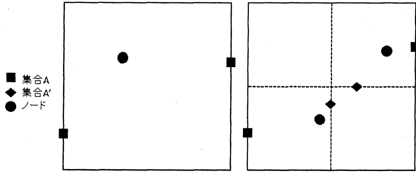
図3 部分解について
