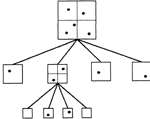
図 4 有向木 B の例
