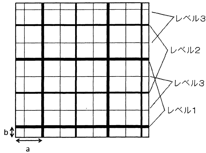
図1 シフトしたグリッド G_i^{(a,b)}
