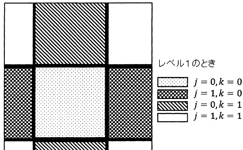
図2 連結でない領域の例
