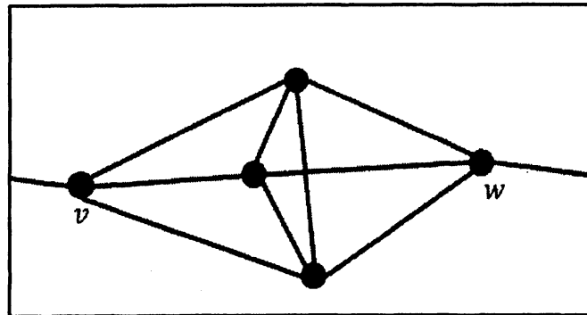
図 6 G と l の交差が辺 e_{vw} との一回のみの例
