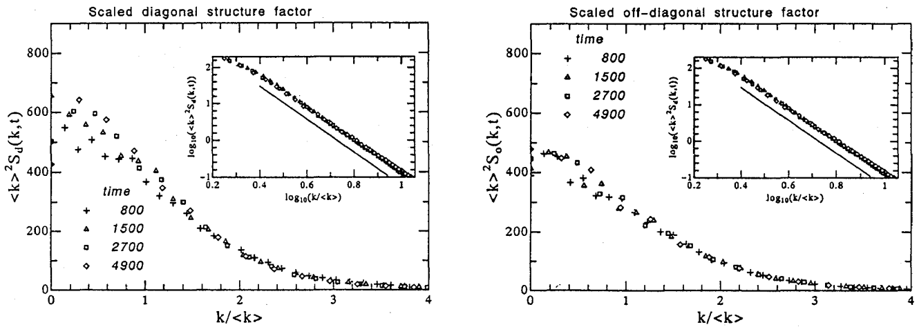
図 3: スケールされた構造因子. 挿入図における実線は傾き -4.5 を表す.
