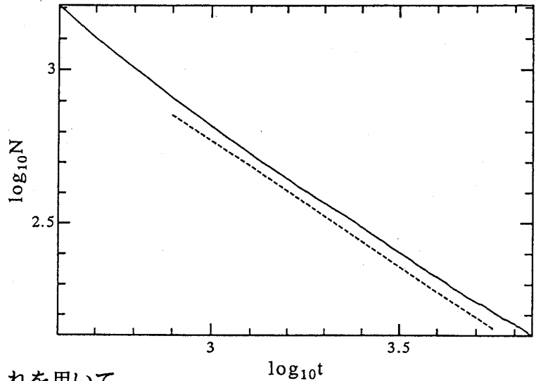
図 2: 欠陥数の時間変化. 破線は傾き -0.92 を表す.
