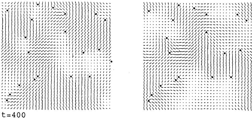
図 1: 配向子と欠陥の分布の一例。左右の図はそれぞれ XY 成分と XZ 成分。
