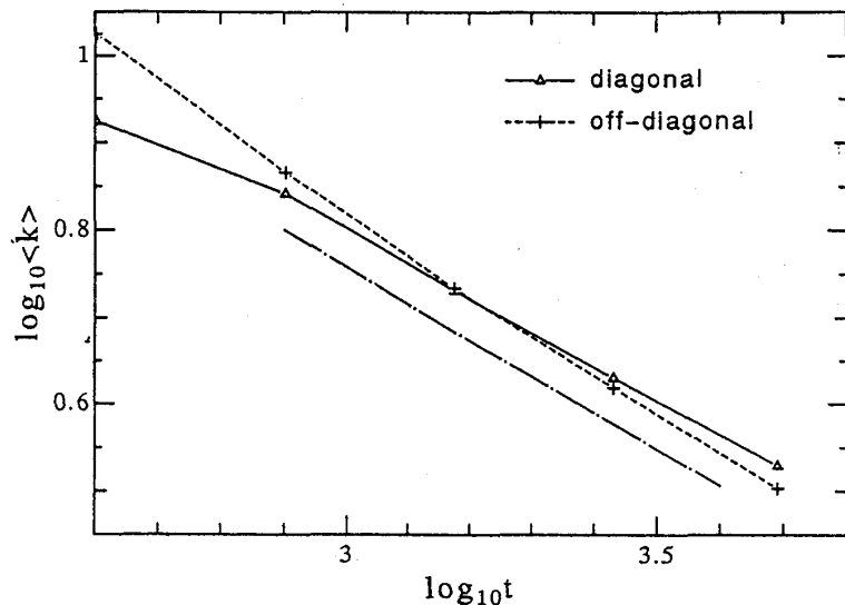
図 4: \langle k \rangle の時間変化. 一点鎖線は傾き -0.42 を表す.
