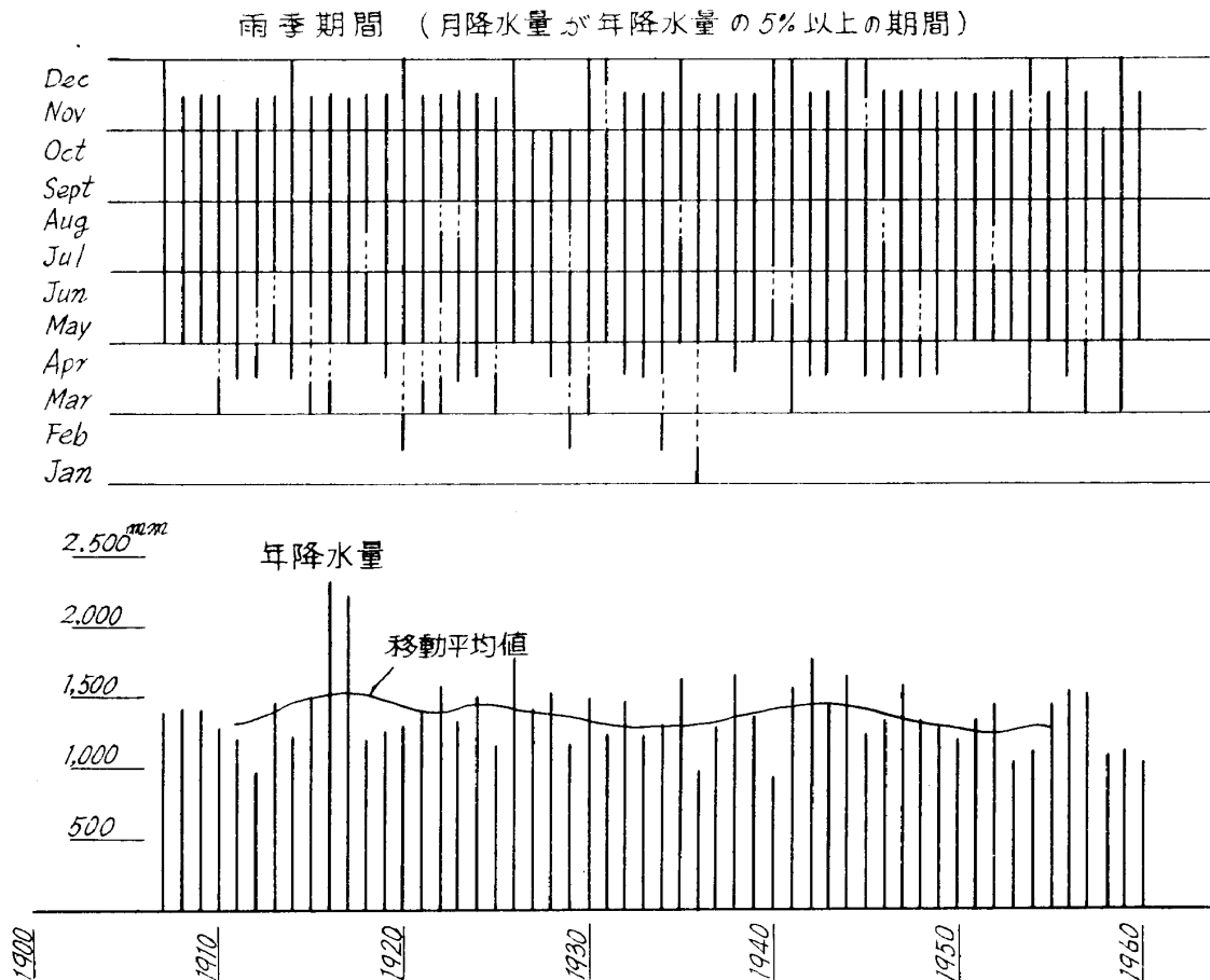
図-3 Phnom Penh における降雨状況
