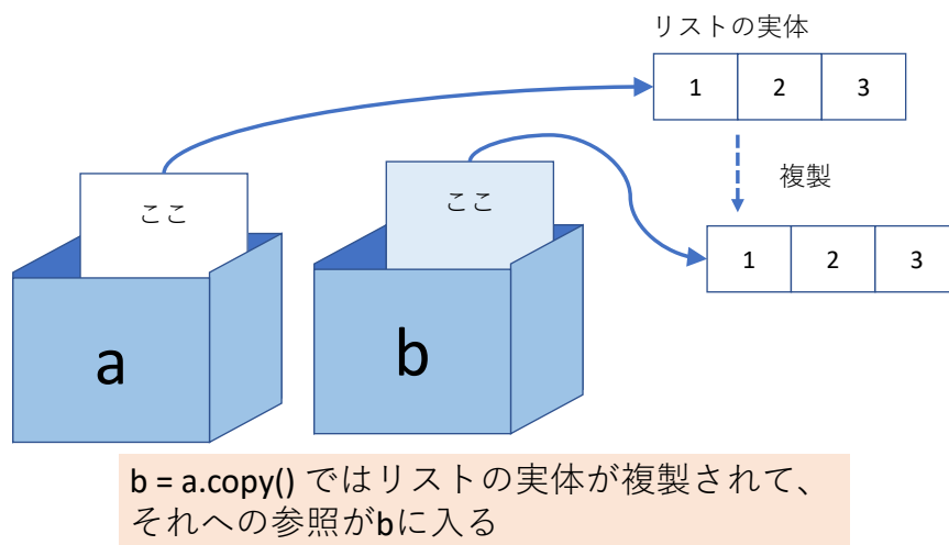
図 4-2 リストのコピー作成と代入
