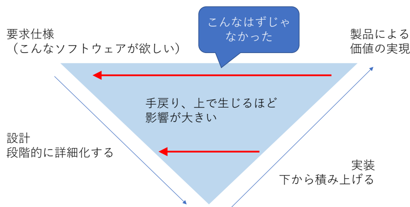
図 13-5 ソフトウェア開発の V モデル
