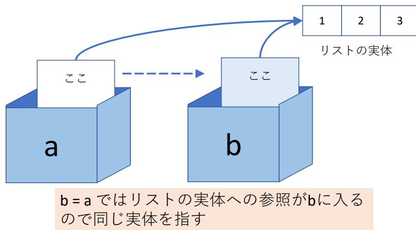
図 4-1 リストの代入
