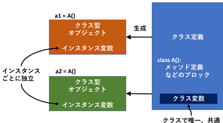
図 11-1 クラス変数とインスタンス変数
