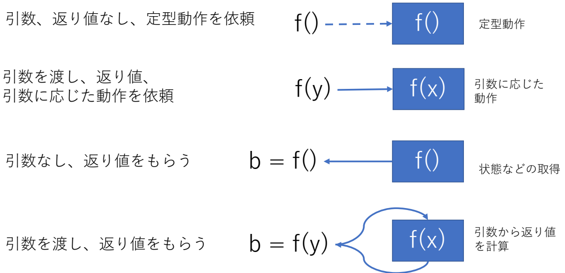
図 7-3 関数の利用パターン
