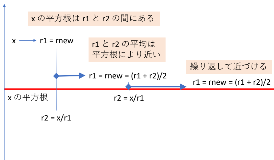
図 3-4 平方根の近似計算の直感的説明
