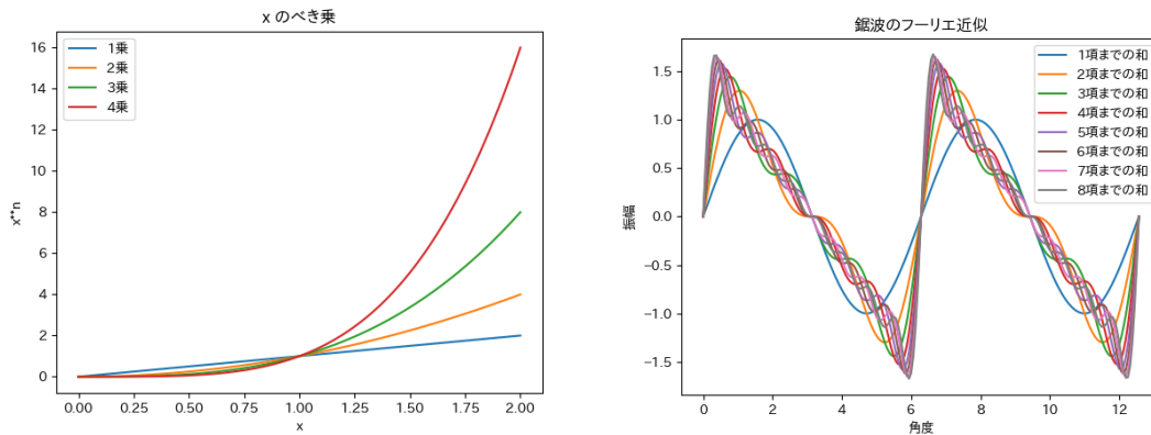
図 14-7 べき乗のグラフとのかぎり波の三角関数の和での近似
