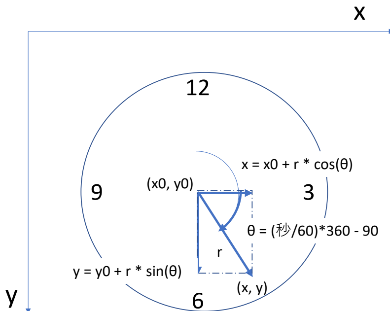
図 10-3 時計の針先位置の計算
