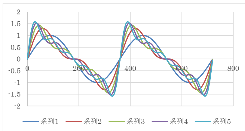
図 12-1 のこぎり波の三角関数の和での近似
