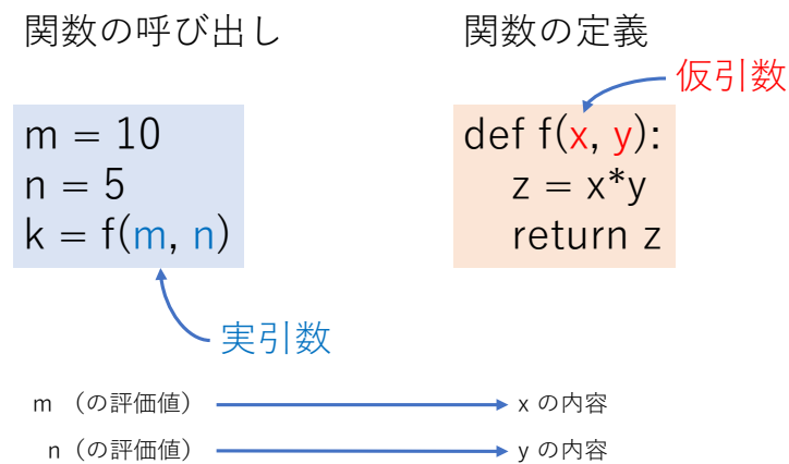
図 7-1 実引数と仮引数
