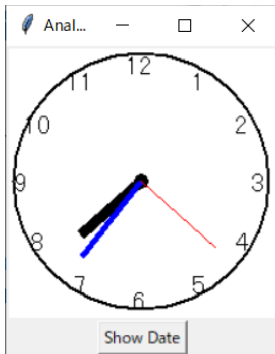
図 10-2 作成するアナログ時計
