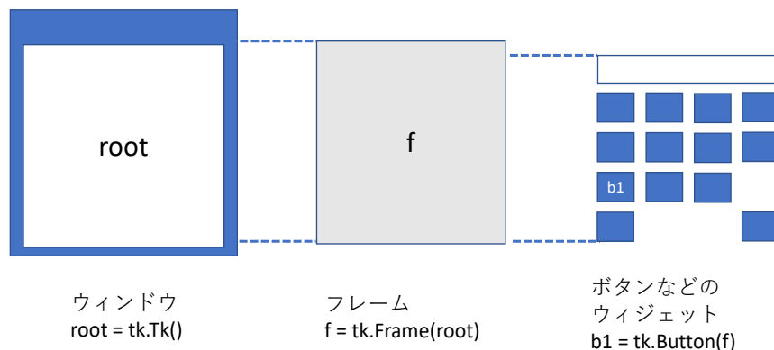
図 9-4 tkinter のオブジェクトの関係
