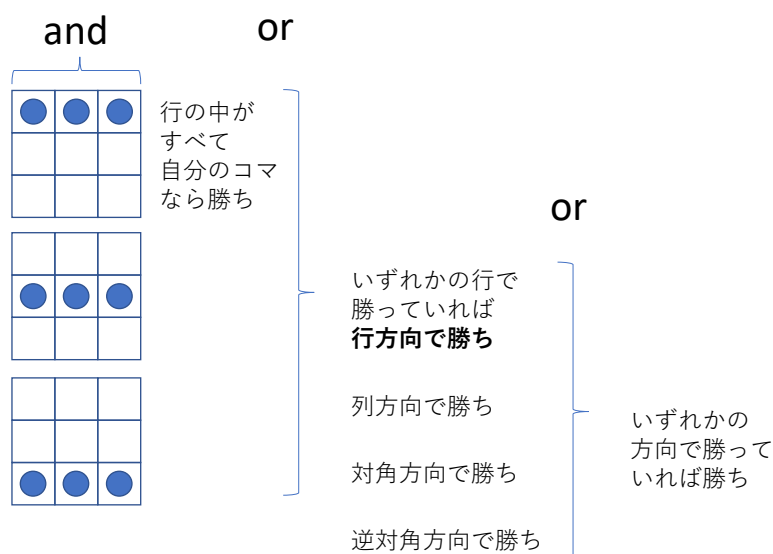
図 13-2 着目する手番の勝ち判定
