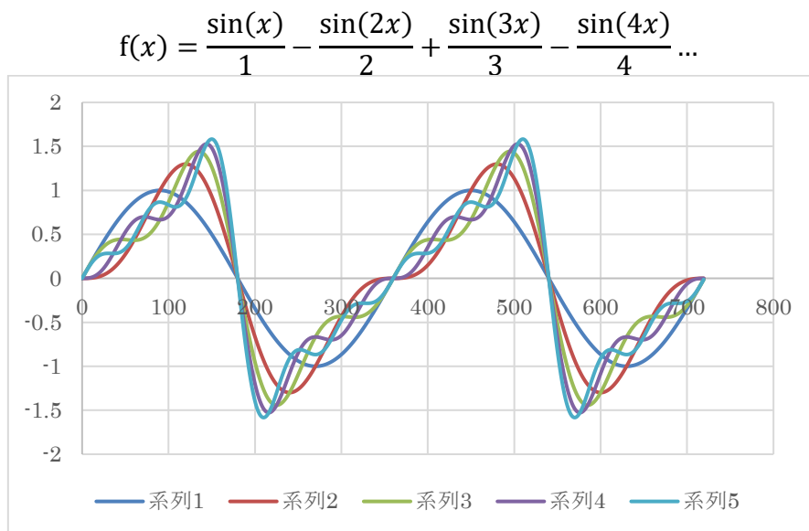
図 12-2 のこぎり波の三角関数の和での近似（原点で傾きが正の場合）
