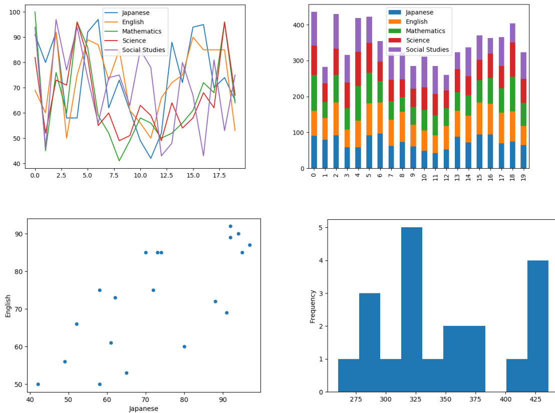
図 14-6 pandas でのグラフ作成
