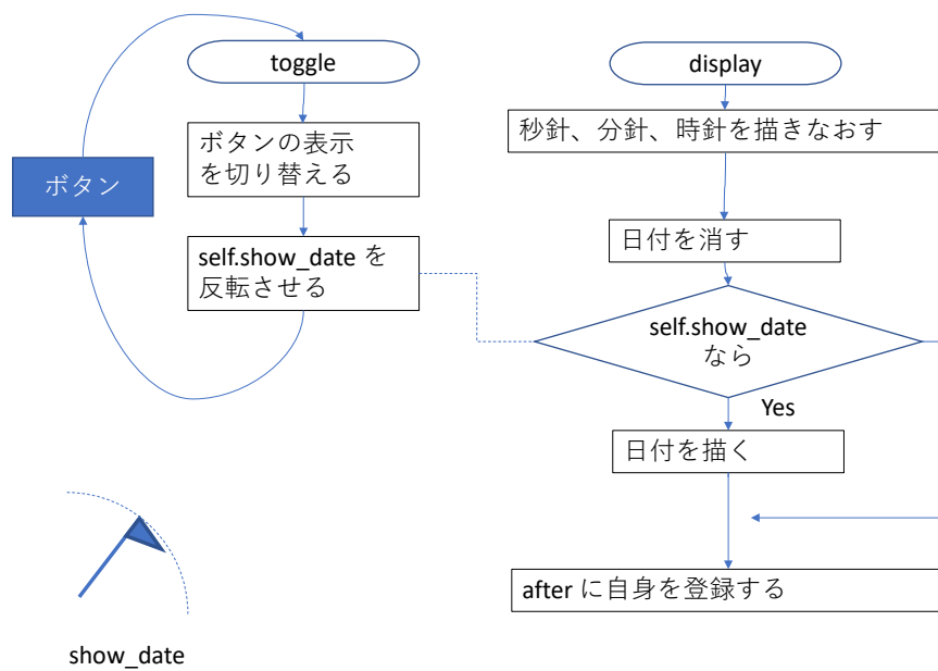
図 10-4 変数を介した動作の協調
