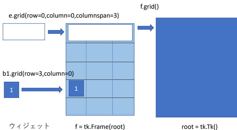
図 9-5 grid によるレイアウト
