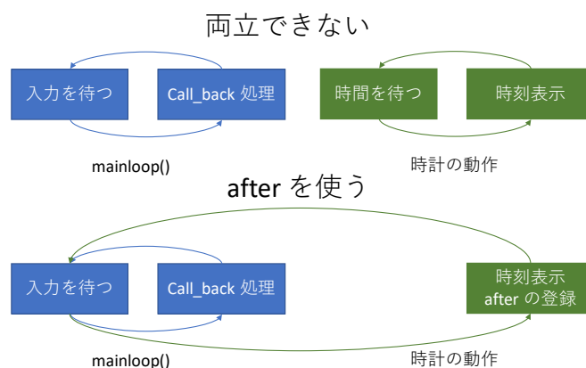
図 10-1 tkinter での after の利用
