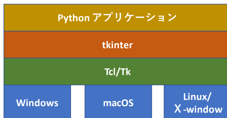
図 9-3 Tkinter のシステム構成
